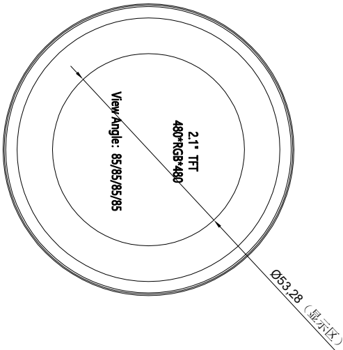
正视图
