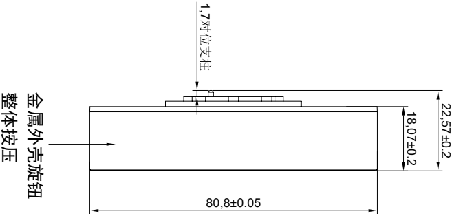
侧视图
